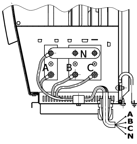
б) Электромонтаж ЭКП
