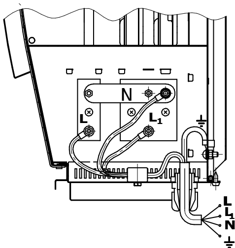
а) Электромонтаж ЭКП
